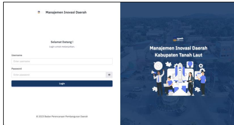
Gambar 3. 1 Halaman Login
